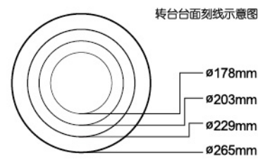
SN4149 蛋糕转台(硬膜) 圆径300x135mm
