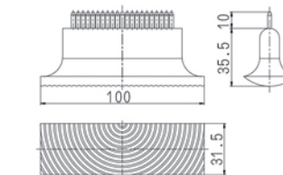
SN3032 木轮根(小) 长度100
