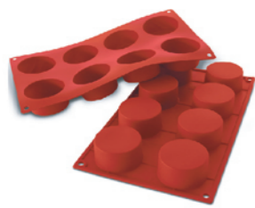
SF028 8连布丁模 295x175x35 单个圆径60 h35 体积约: 90ml
