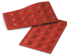
SF031 15连贝壳模 295x175x10 单个44x34 h10 体积约: 10ml
