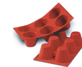
SF052 6连布丁模 295x175x60 单个圆径75 h60 体积约: 165ml
