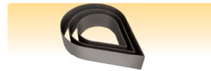
SN3905 6"水滴型圈(硬膜) 152x108x50 SN3906 8"水滴型圈(硬膜) 203x144x50 SN3907 10"水滴型圈(硬膜) 254x179x55
